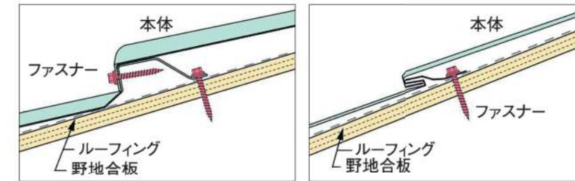
従来のインターロック工法
